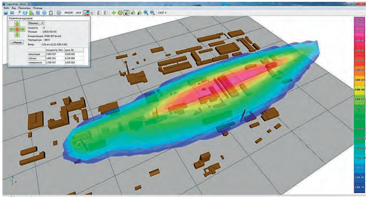
Рис. 4 – Моделирование процессов переноса и осаждения радионуклидов в условиях зданий и сооружений промплощадки ЯРОО
