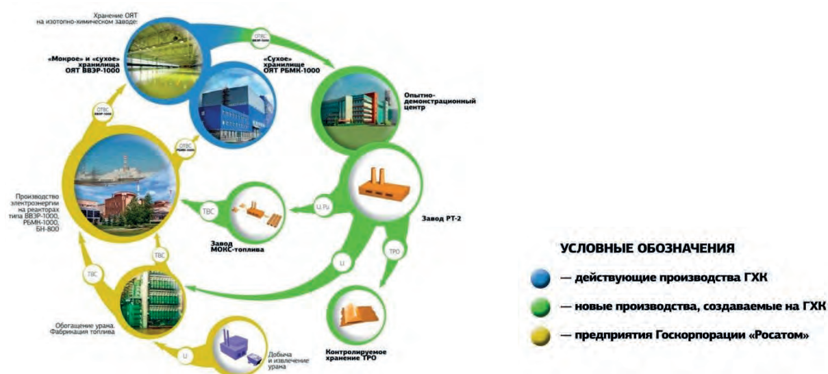
Рис. 1 – Концепция замыкания ядерного топливного цикла на ФГУП «ГХК»
