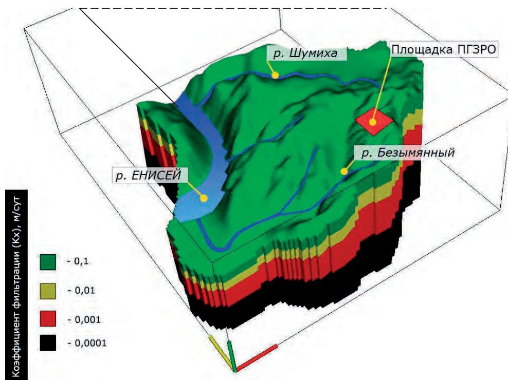
Рис. 4 - Концептуальная схема 3D гидрогеологической модели
