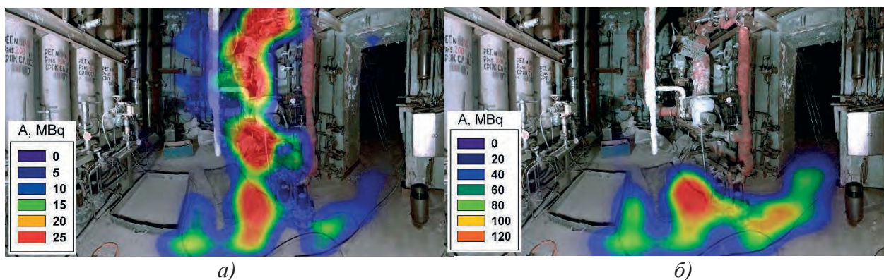
Рис. 1 – Распределение активности Cs-137 (а) и Co-60 (б) в помещении петлевой установки ПВК
