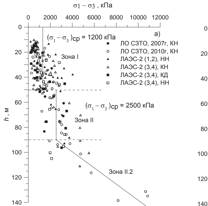
Рис. 2 - График зависимости разности осевых разрушающих и объемных напряжений q_p = \sigma_1^p - \sigma_3^p от глубины отбора образца. Обобщенные данные КД, КН и НН испытаний
