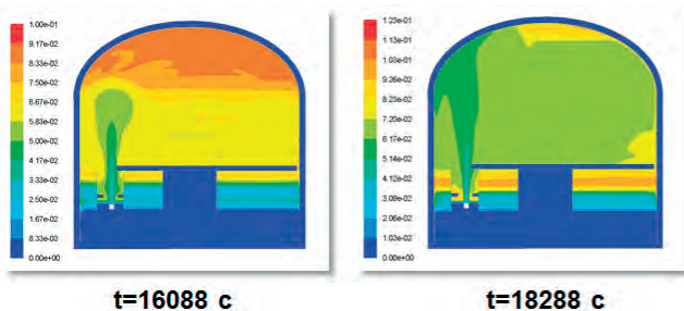
Рис. 3 – Стратификация в аппаратном зале при выходе основной массы водорода
