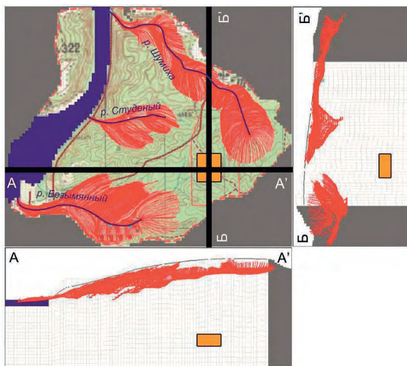
Рис. 5 - Зоны захвата инфильтрационных вод поверхностными водотоками (прямоугольник – условный контур объекта)
