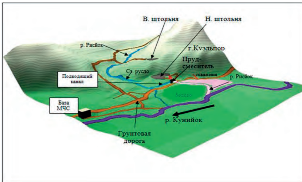
Рис. 3 – МЯВ «Днепр 1, 2». Схема разбавления трития после выноса с шахтными водами
