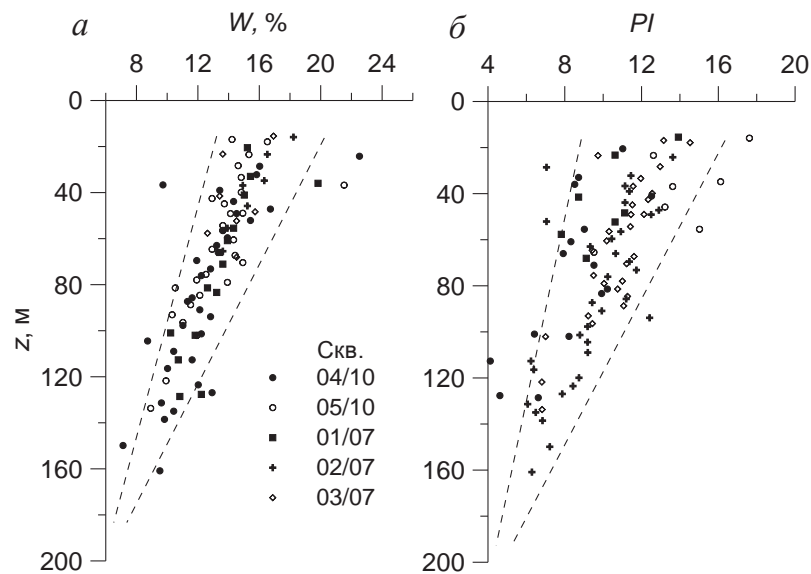
Рис. 1 - Изменение влажности (а), числа пластичности (б), с глубиной (глины Vkt)
