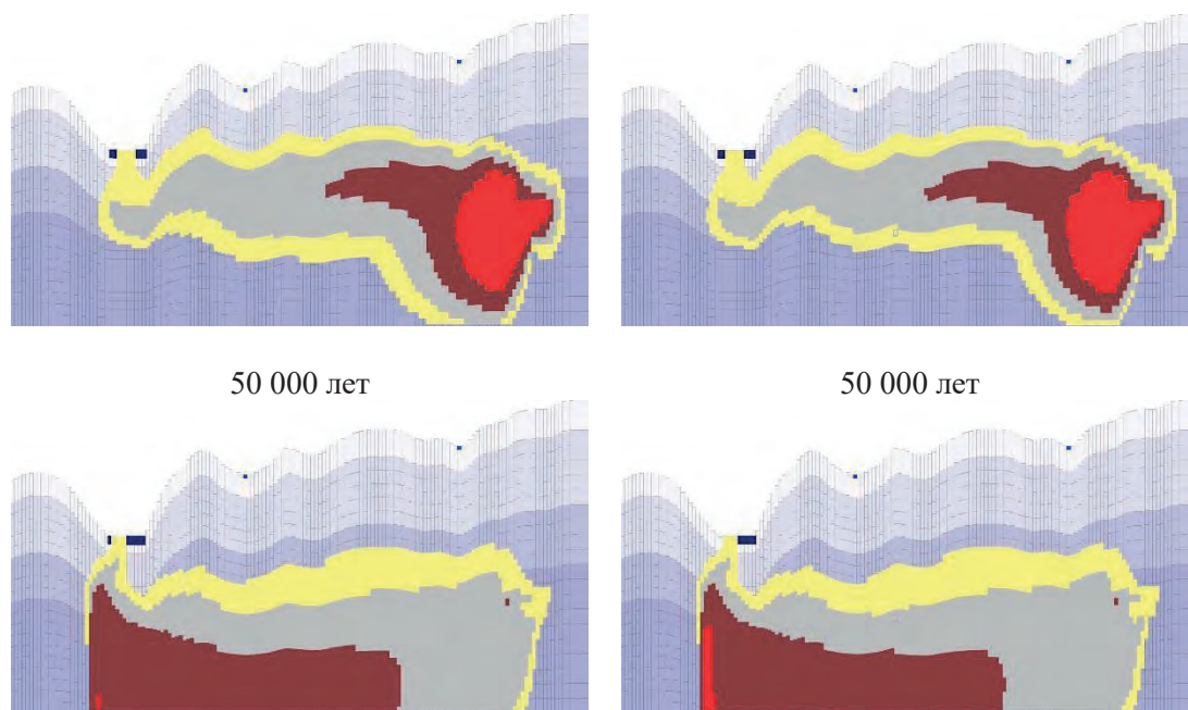
Рис. 6 - Конфигурация ореола загрязнения I-129 в относительных концентрациях; время указано с момента выхода за пределы СИБ; фон - зоны фильтрационной неоднородности
