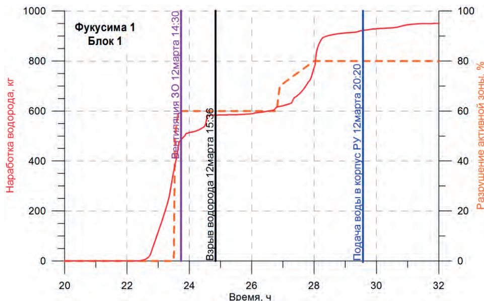
Рис. 5 – Оценка времени взрыва водорода на АЭС Фукусима-1
