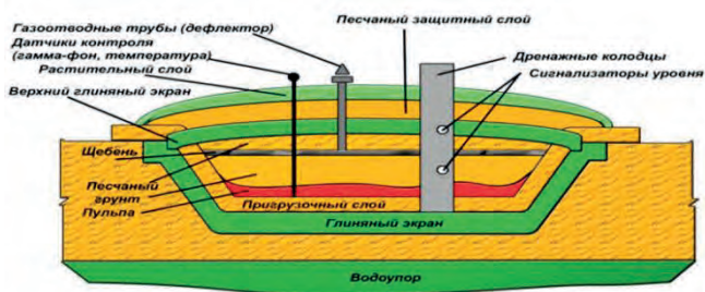
Рис. 10 – Схема барьеров безопасности Б-2
