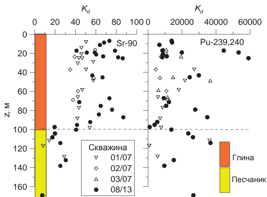
Рис. 3 - Пример изменения коэффициента K_d ( \text{см}^3/\text{г} ), характеризующего сорбцию Sr-90 и Pu-239, 240, по мощности. Значки отвечают различным скважинам
