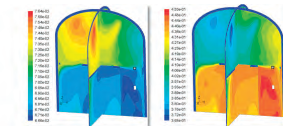
Рис. 4 – Распределение водорода и пара: 1360 с
