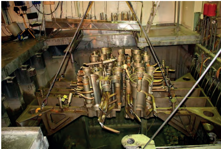
Рис. 6 – Удаление опорной решетки реактора МР
