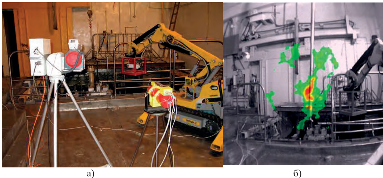
Рис. 3 – Процесс измерения распределения активности вдоль петлевого канала (а) и полученные результаты (б)
