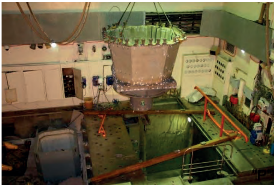
Рис. 7 – Демонтаж корпуса реактора МР
