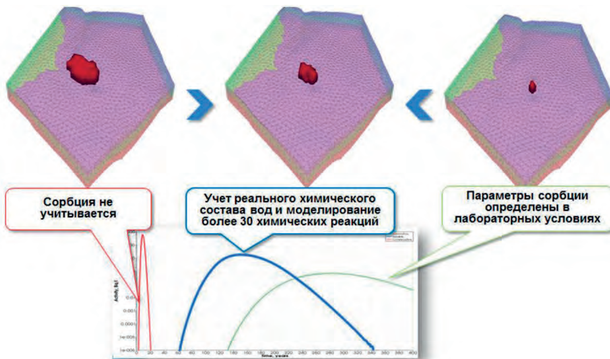
Рис. 7 – Моделирование геомиграции в связке GeRa+PHREEQC
